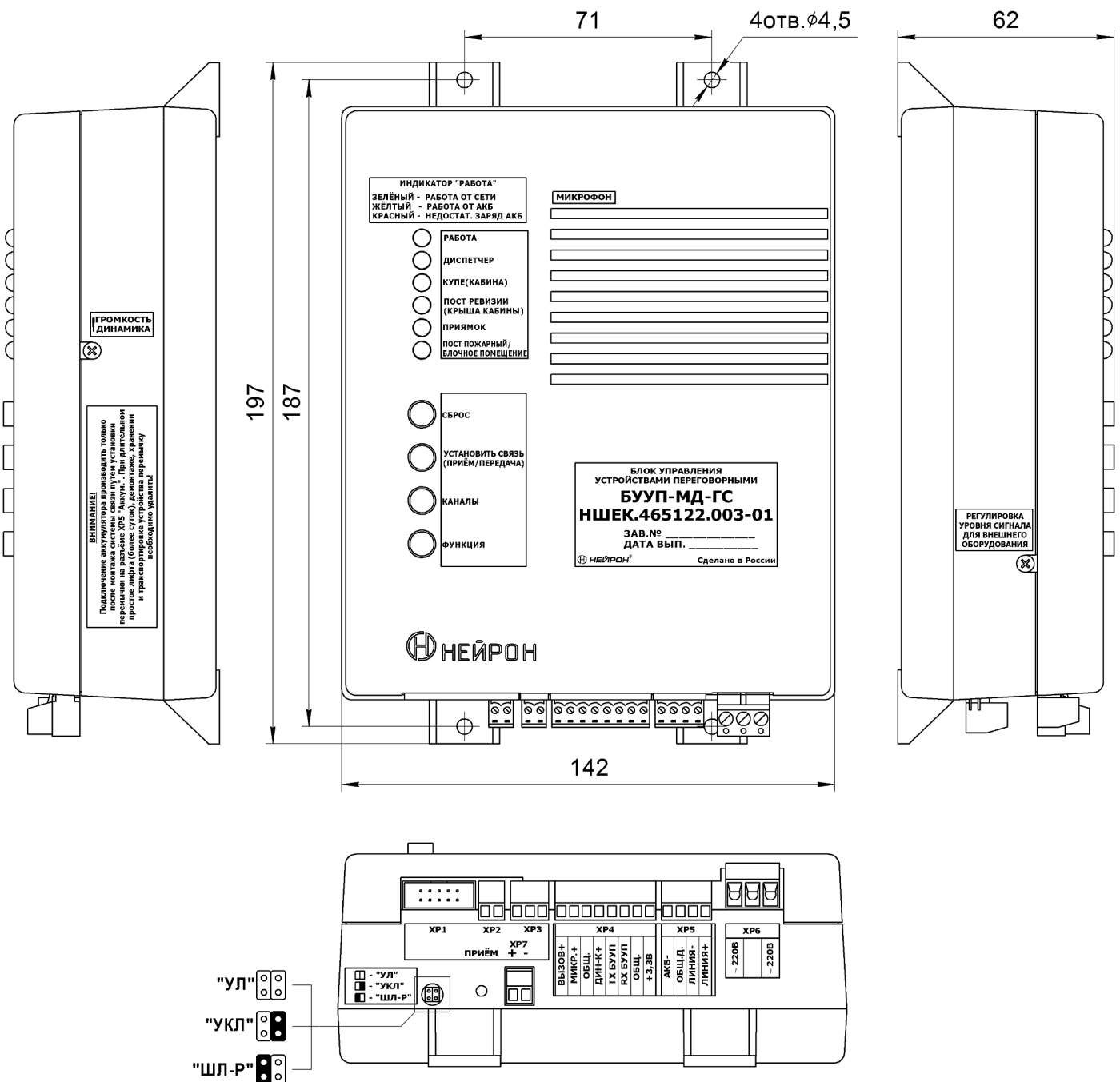
Рис.1 Внешний вид Блока управления устройствами переговорными «БУУП-МД-ГС» НШЕК.465122.003-01
